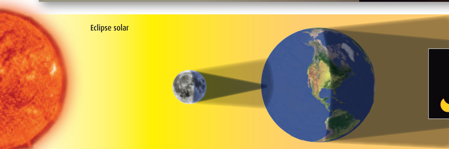
Eclipse total de sol.
