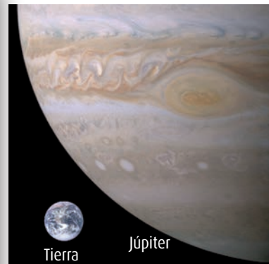
Comparación del tamaño de un planeta interior y uno exterior.
