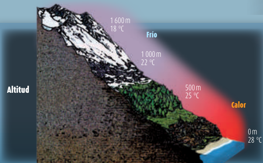
El relieve, el viento y la humedad son algunos de los elementos modificadores del clima.
